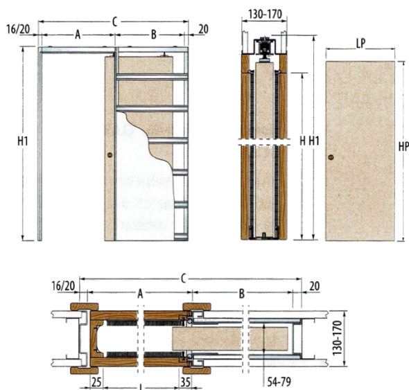
SYSTEM PRZESUWNY WEWNĘTRZNY POJEDYNCZY
