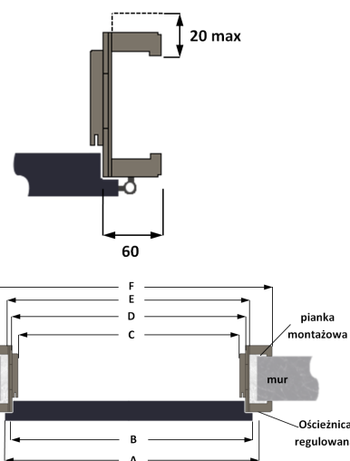
OŚCIEŻNICA REGULOWANA
