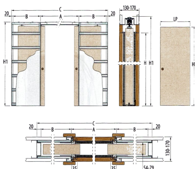
SYSTEM PRZESUWNY WEWNĘTRZNY PODWÓJNY
